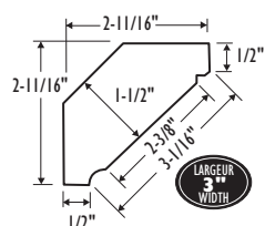
F Raccord de corniches pour des moulures d'une hauteur inférieure à 2 3/4"
