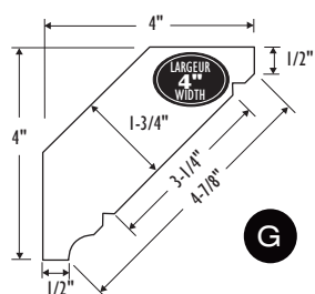
G Raccord de corniches pour des moulures d'une hauteur inférieure à 4 5/8"
